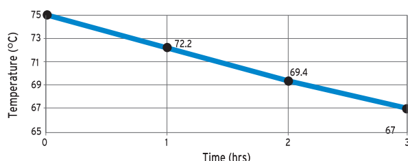
Cooling Chart / Diagramme de Refroidissement
